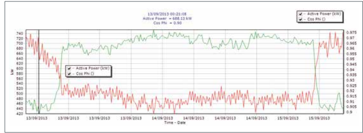
Fig. 2: Relatório de contagem do contador principal da fábrica. O consumo de electricidade (potência activa) e o respectivo factor de potência (cos phi) são registados em intervalos de 15 minutos. Durante o fim-de-semana apenas algumas máquinas estão a produzir e como resultado a potência activa diminui e o factor de potência melhora. O gráfico mostra que o factor de potência permanece sempre acima de 0,9, o que indica uma situação aceitável. Este gráfico também permite avaliar o funcionamento das baterias de condensadores para melhorar o factor de potência.
