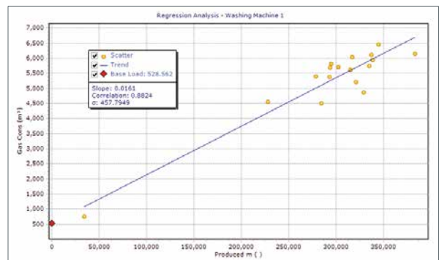
Fig. 7: Linha Característica de Performance (PCL).
